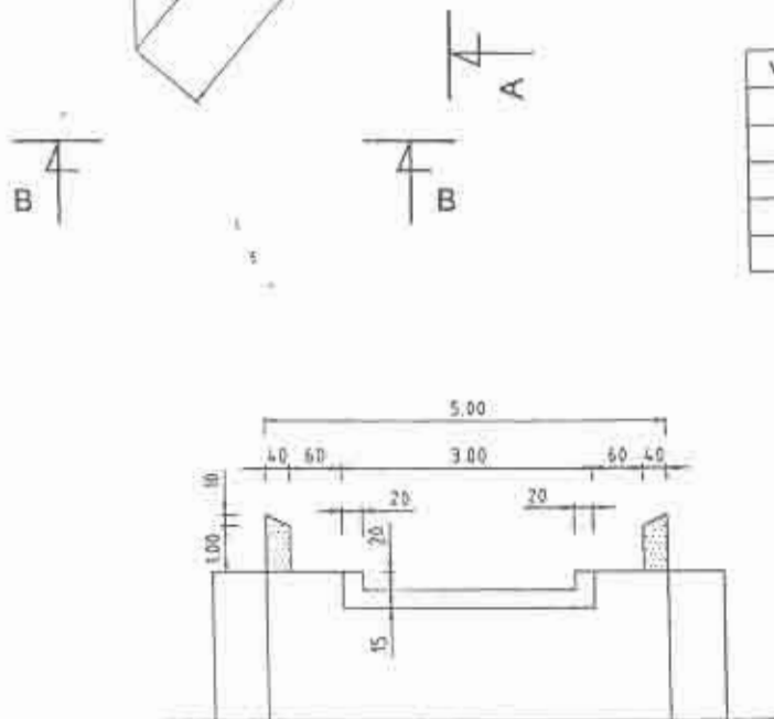
COUPE A-A
